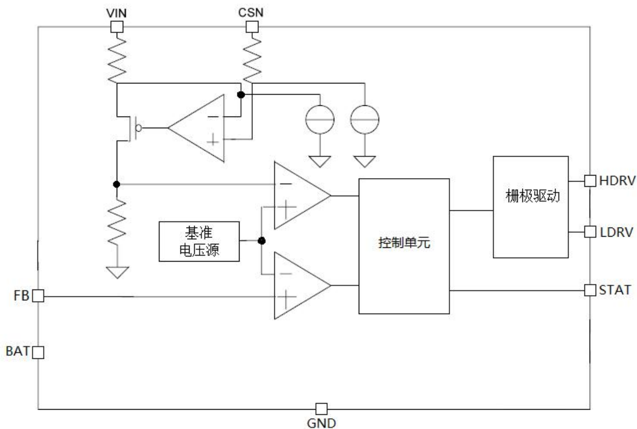
图 3 功能框图
