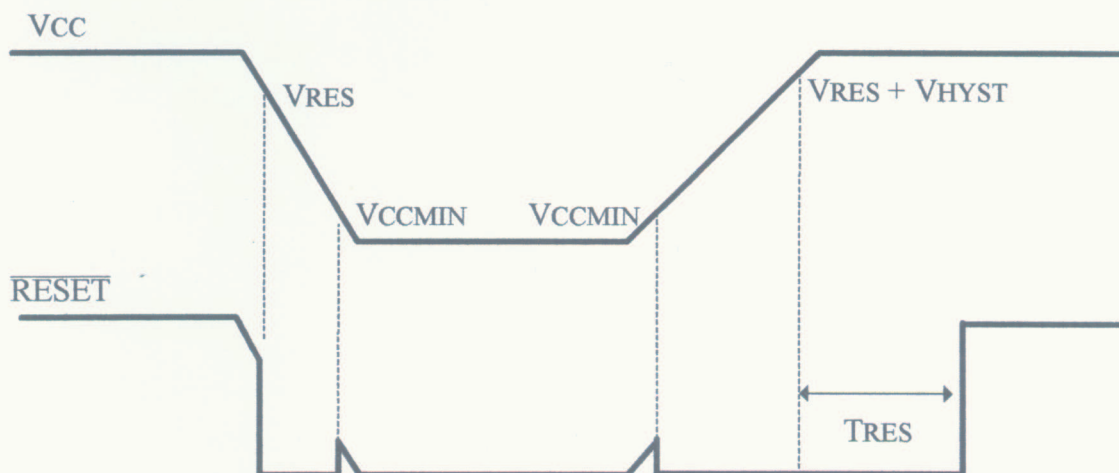
图2 时序图
