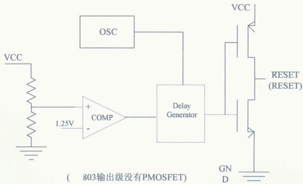
图1 功能框图
