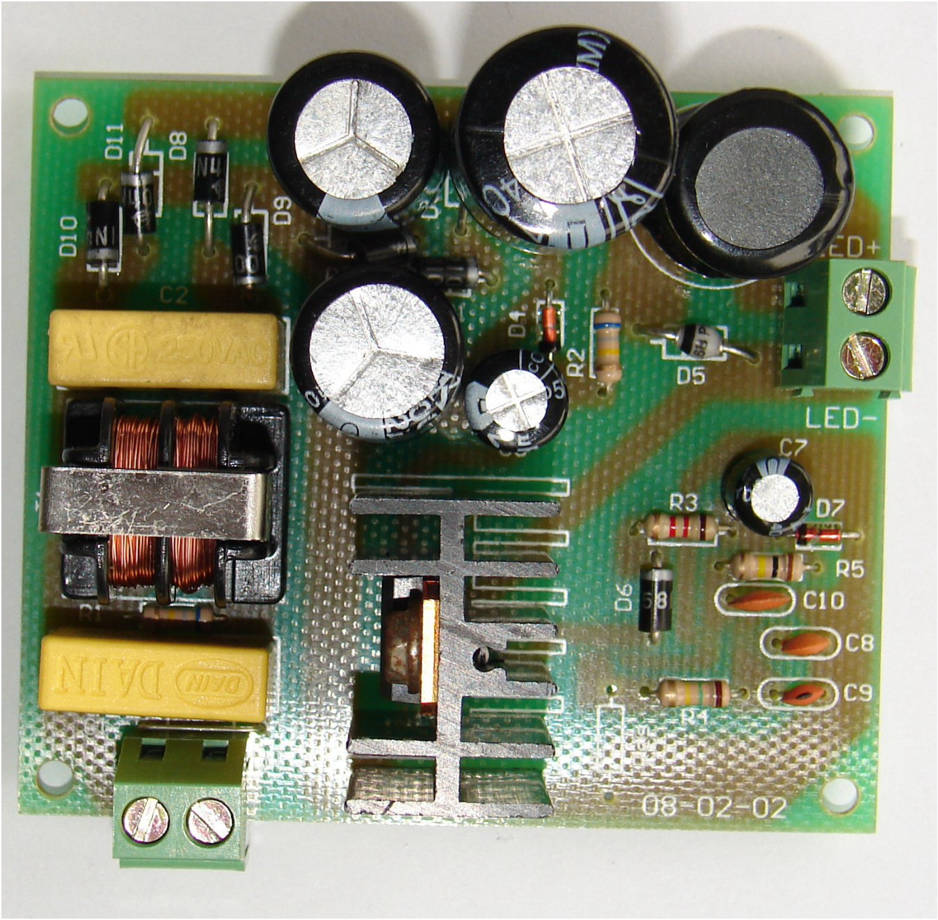
图 4 图 3 电路制作的电路板
